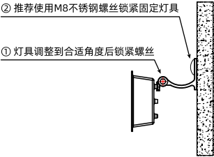
侧面安装示意图
