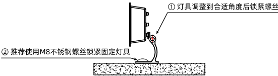
底部安装示意图
