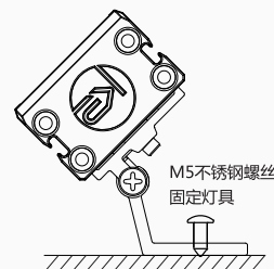
底部安装示意图
