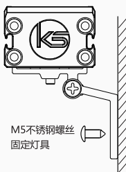
侧面安装示意图
