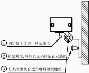
侧面安装示意图
